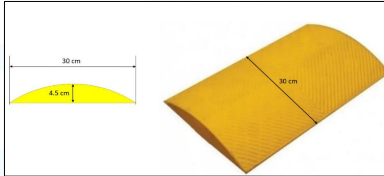
Şekil 2. Yarış Pistinde Kullanılan Kasis
